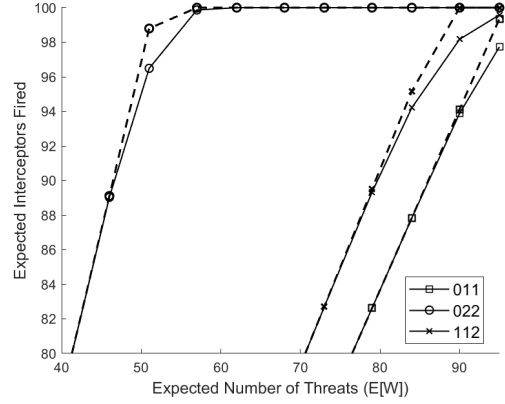
(d) Expected Number of Interceptors, p = 0.9
