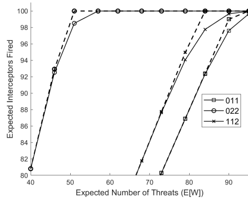
(d) Expected Number of Interceptors, p = 0.9
